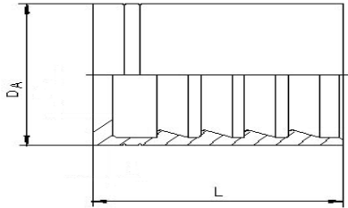
Bucșă compactă pentru furtun nedecojit 1SN/2SN
