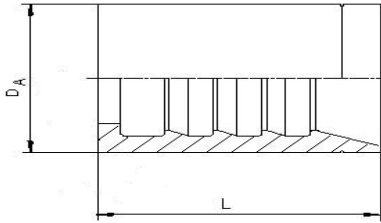
Bucșă pentru furtun decojit 1 SN/1 ST
