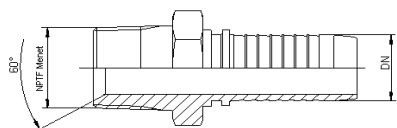
( AGN ) Armătură cu filet exterior în țol NPT cu con
