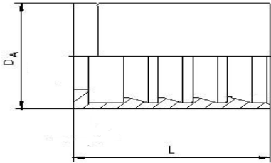
Bucșă pentru furtun nedecojit 1 SN
