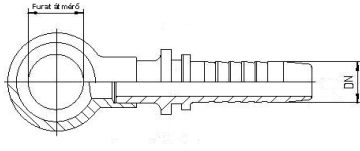
(RNM) Armătură tip inel pentru șurub cu filet metric
