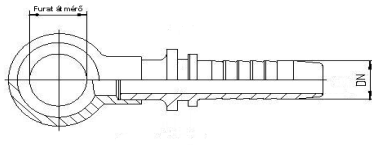
(RGM) Armătură tip inel pentru șurub cu filet BSP
