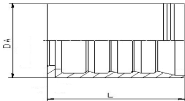
Bucșă pentru furtun decojit 4 SP
