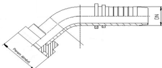
( CAT ) Armătură cu flanșă CATERPILLAR la 45°
