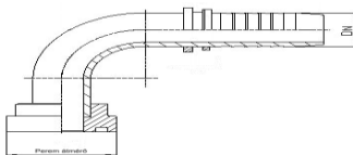
( CAT ) Armătură cu flanșă CATERPILLAR la 90°
