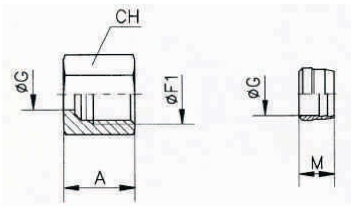
Olandeză si inel tăietor TN81 - TN88
